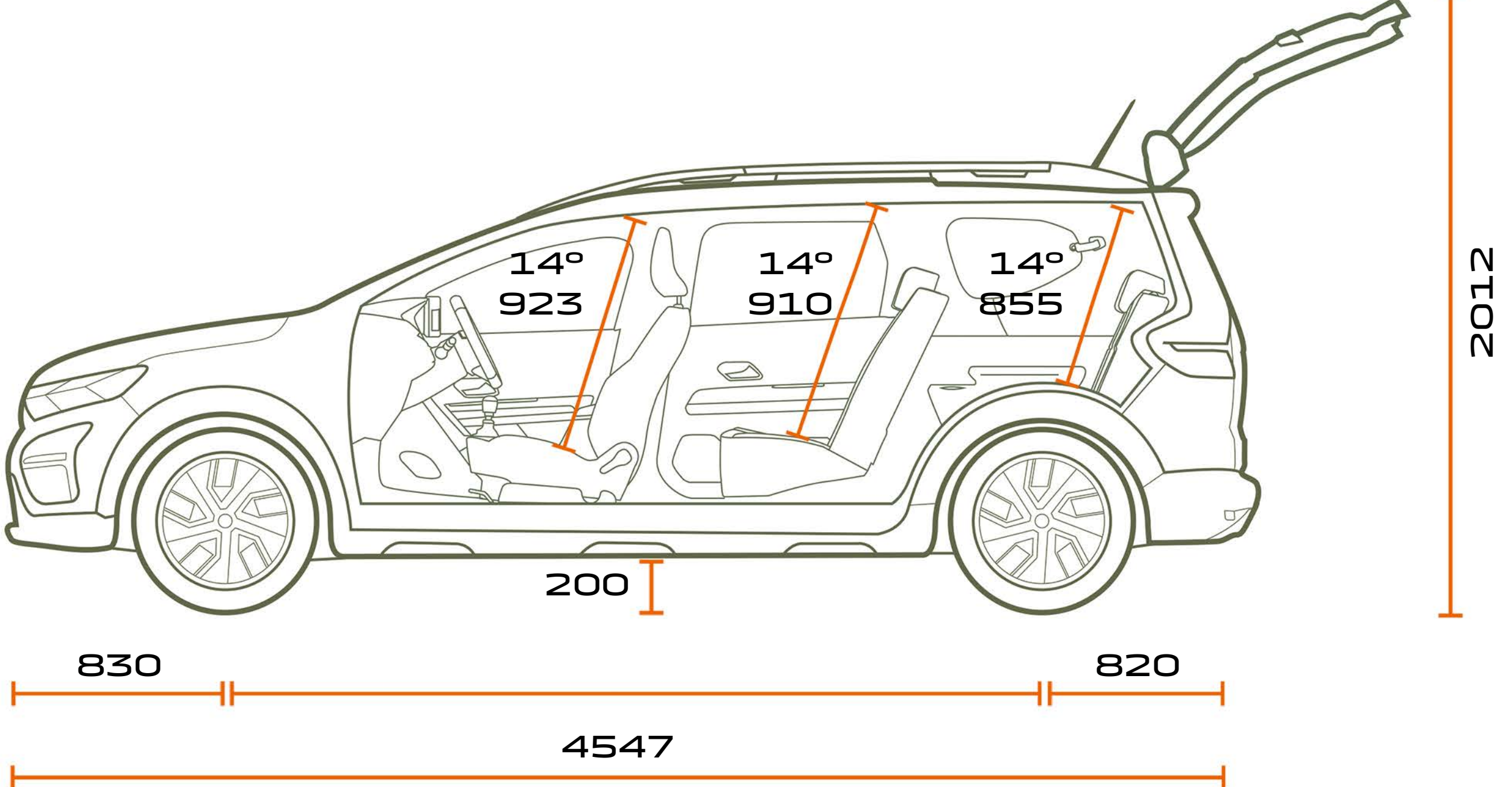
7 VIETŲ VARIANTAS IŠ ŠONO
