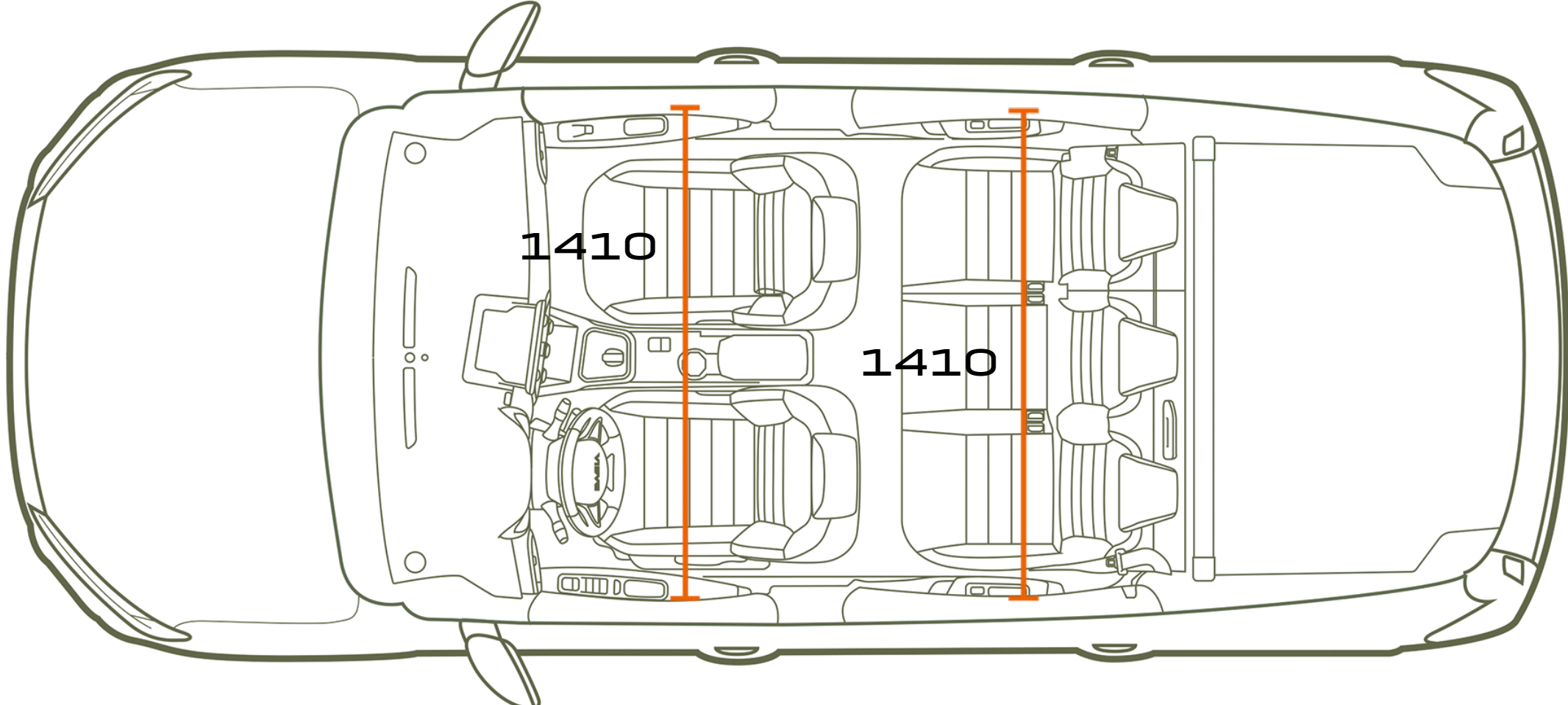
5 VIETŲ VARIANTAS IŠ VIRŠAUS
