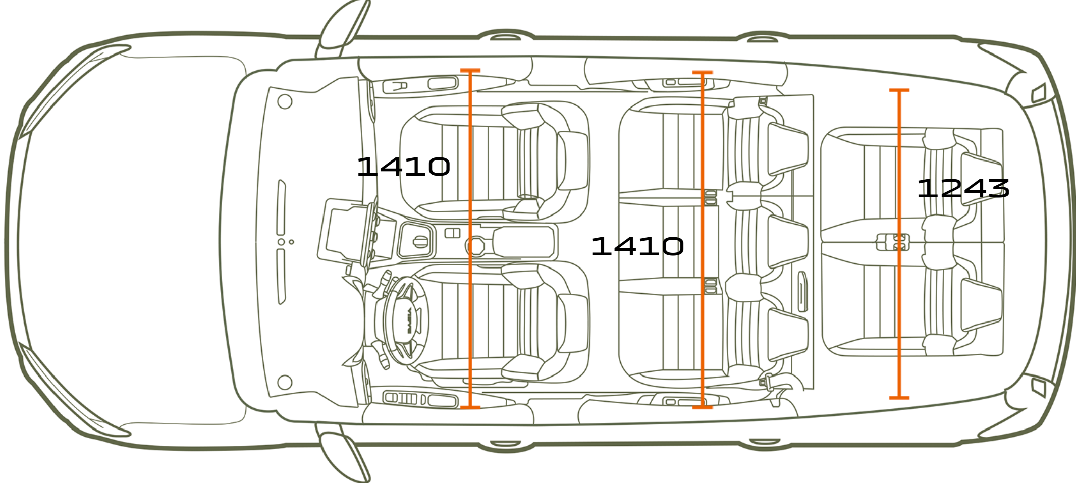
7 VIETŲ VARIANTAS IŠ VIRŠAUS
